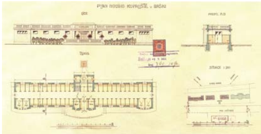
Matěj Blecha, Baška, kupalište, projekt
