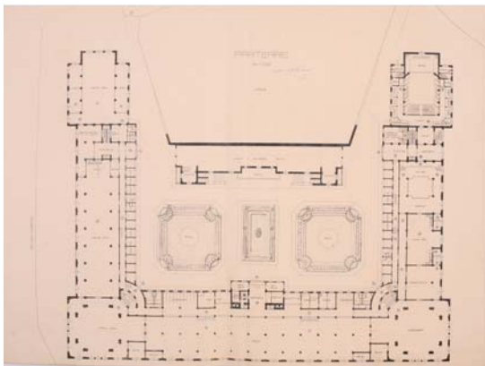
Adolf Loos, Opatija, hotel, tlocrt
